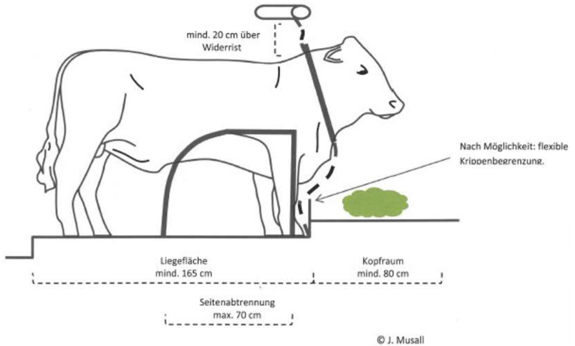
Abbildung: Mindestabmessungen für die Anbindehaltung von Rindern
